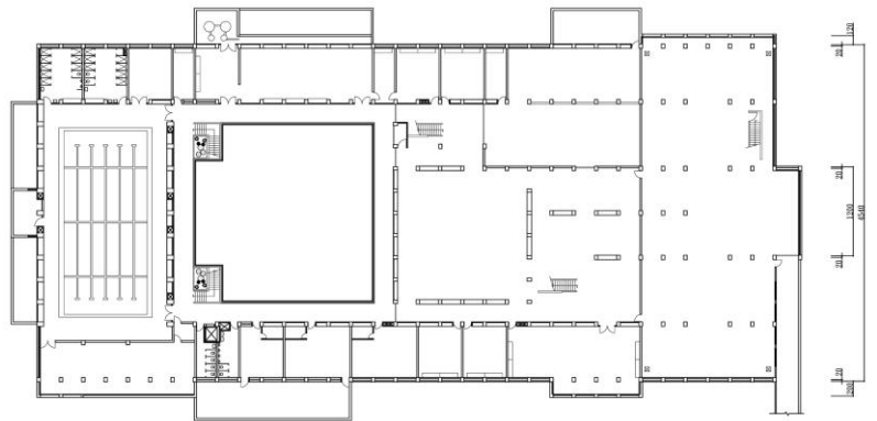
地下平面圖 S= 1/200
